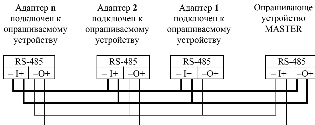
Рисунок 2 - Схема многоточечного соединения
